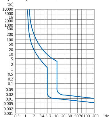
Характеристика С
